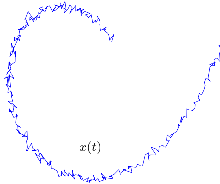
Figura 1.2: Una realización de la solución de una Ecuación Diferencial Estocástica.
