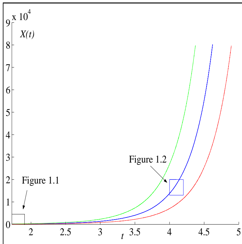
Figura 6.1: Tres trayectorias que explotan
