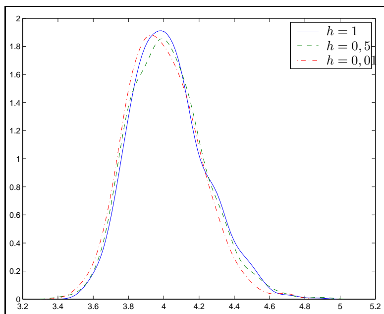
Figura 6.4: Estimación por núcleos de la densidad de \tau para diferentes valores de h
