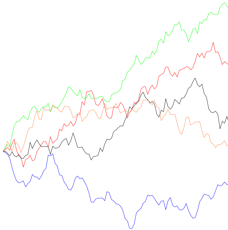
Figura 2.2: Cinco simulaciones de un Movimiento Browniano unidimensional
