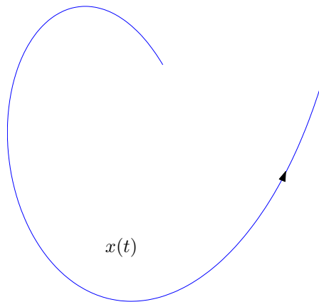
Figura 1.1: Trayectoria de una solución de una EDO
