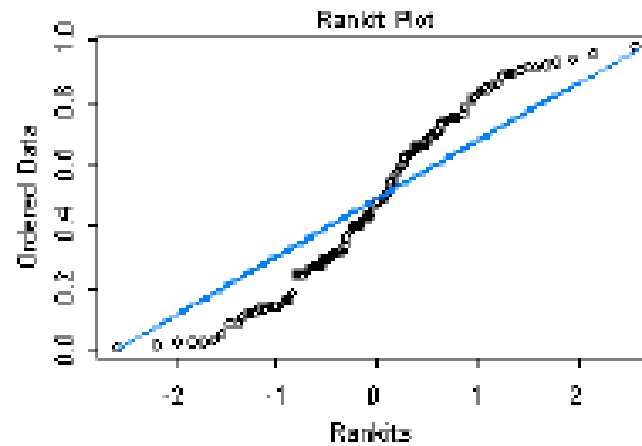
Simétrica con Colas Pesadas
