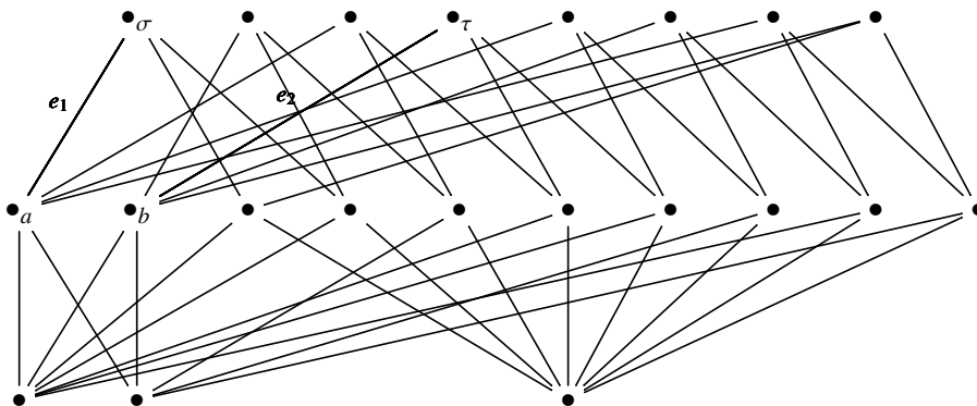
Figure 3.14: Face poset asociado a la estructura h-regular del Pentágono.
