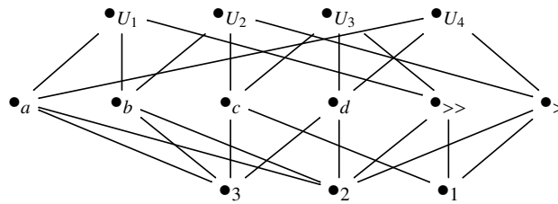
Figure 4.10: El espacio finito \tilde{M}(\mathcal{U}) asociado a un cubrimiento cuasi-bueno \mathcal{U} del Dunce Hat.
