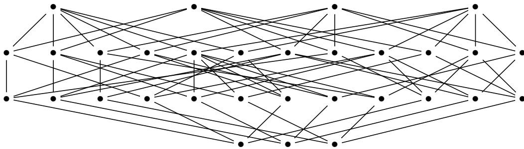
Figure 4.9: El espacio finito M(\mathcal{U}) asociado a un cubrimiento cuasi-bueno del Dunce Hat.
